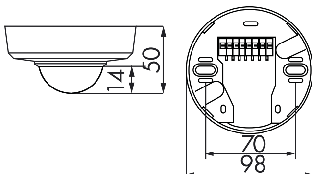
Dimensions 92550
